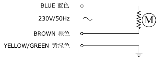
Wiring diagram 接线图
